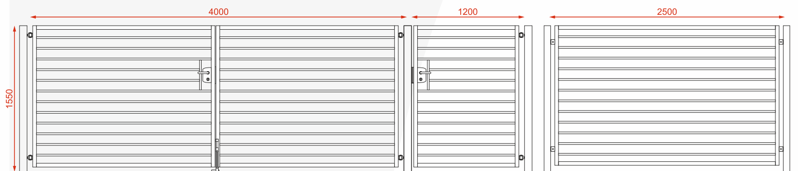
system ogrodzenia palisadowego o spójnym wyglądzie (brama, furtka, przesło ogrodzeniowe) [widok od wewnątrz]
